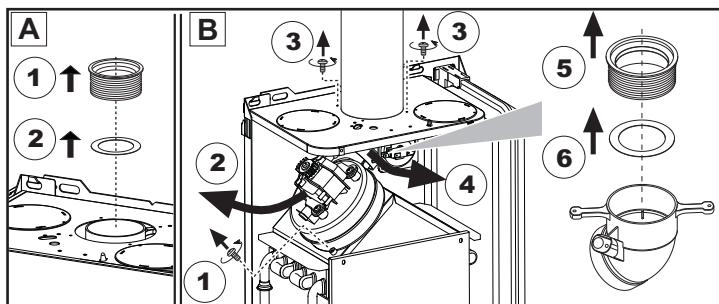
A Sostituzione diaframma con caldaia non installata
