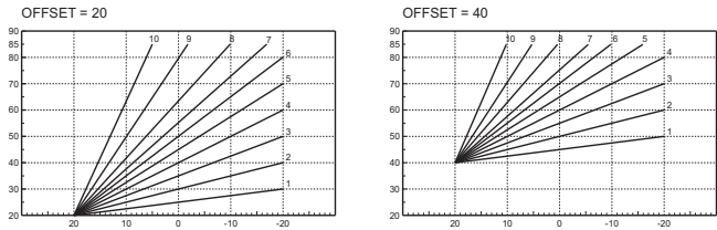
рис. 6 - Пример параллельного смещения компенсационных характеристик
