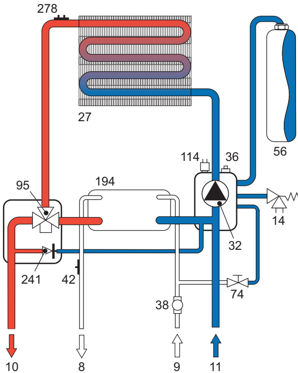
fig. 22 - Circuito de calefacción
