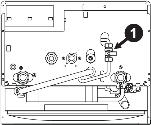
fig. 7 - Filling cock
