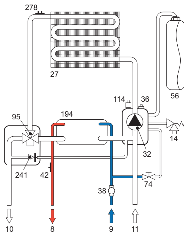
fig. 23 - Circuito sanitario
