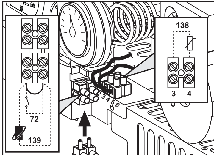
fig. 8 - Accesso alla morsettiera
