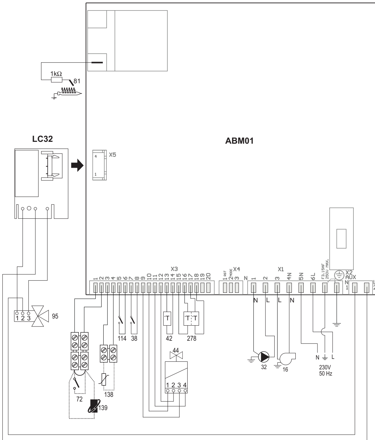
рис. 24 - Электрическая система
