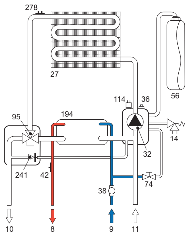
рис. 23 - Контур ГВС
