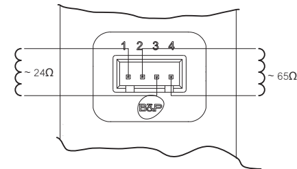
рис. 19 - Электрический разъем для подключения газового клапана
