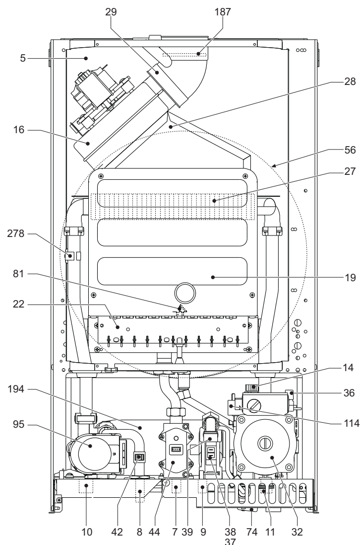
fig. 21 - Vista generale CLIZIA D 24 AS
