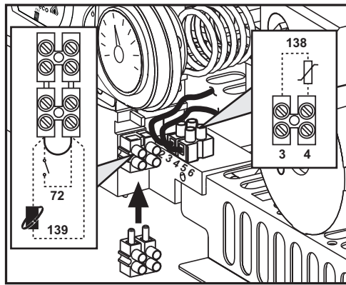
рис. 8 - Доступ к клеммной коробке
