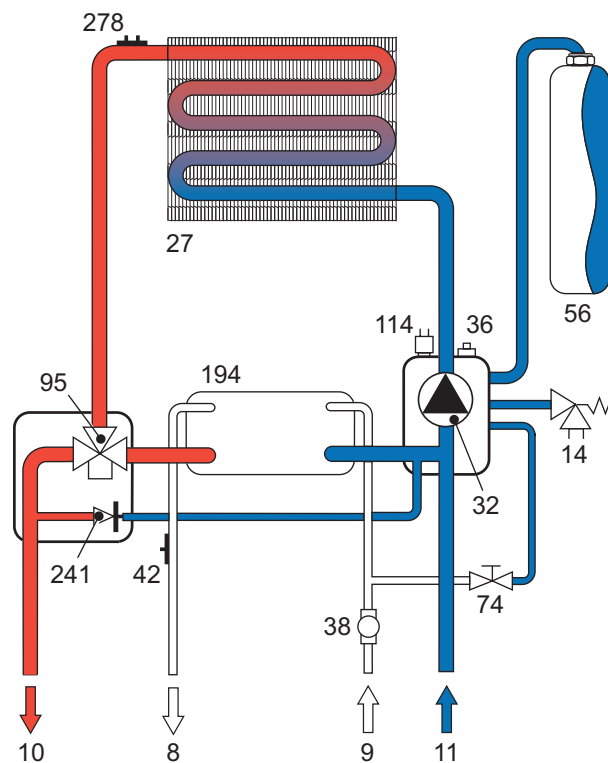
fig. 22 - Circuito riscaldamento
